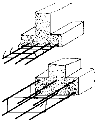
SEMELLE DE FONDATION
