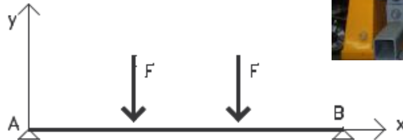
Schéma mécanique
