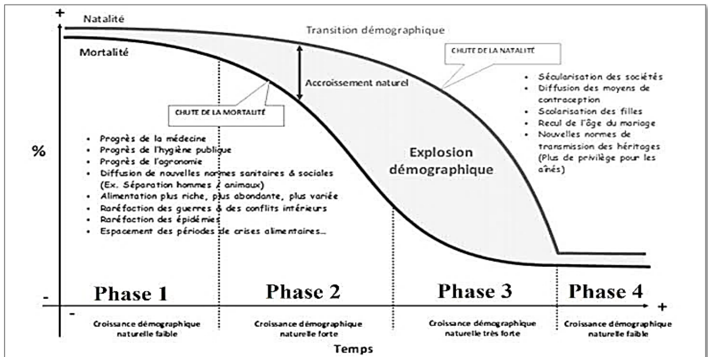
الشكل رقم 01: الشكل الكلاسيكي لنظرية التحول الديموغرافي
