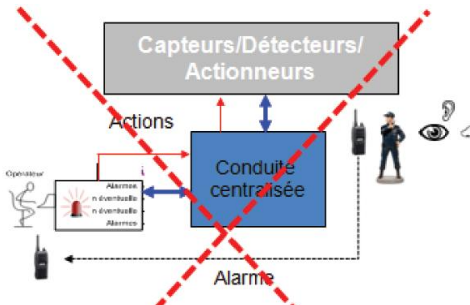
Figure 10. Alarmes indépendantes du système de conduite centralisé.
