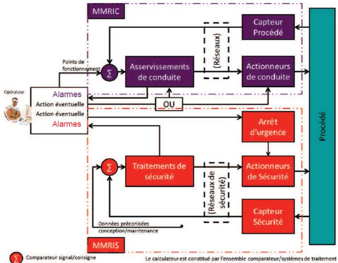
Figure 11. Illustration de la distinction fonctionnelle et matérielle, entre une MMRIC et une MMRIS
