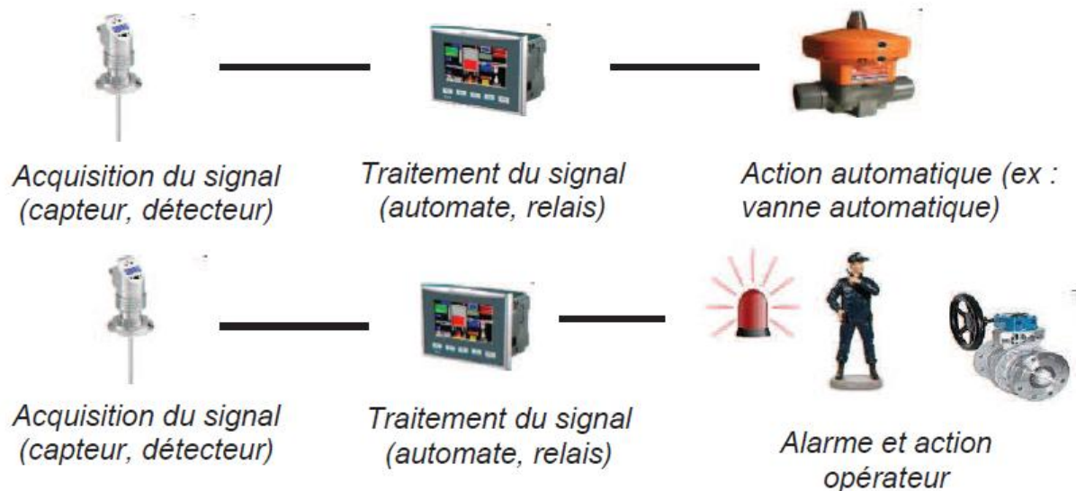
Figure 3. Chaîne instrumentée de MMRI
