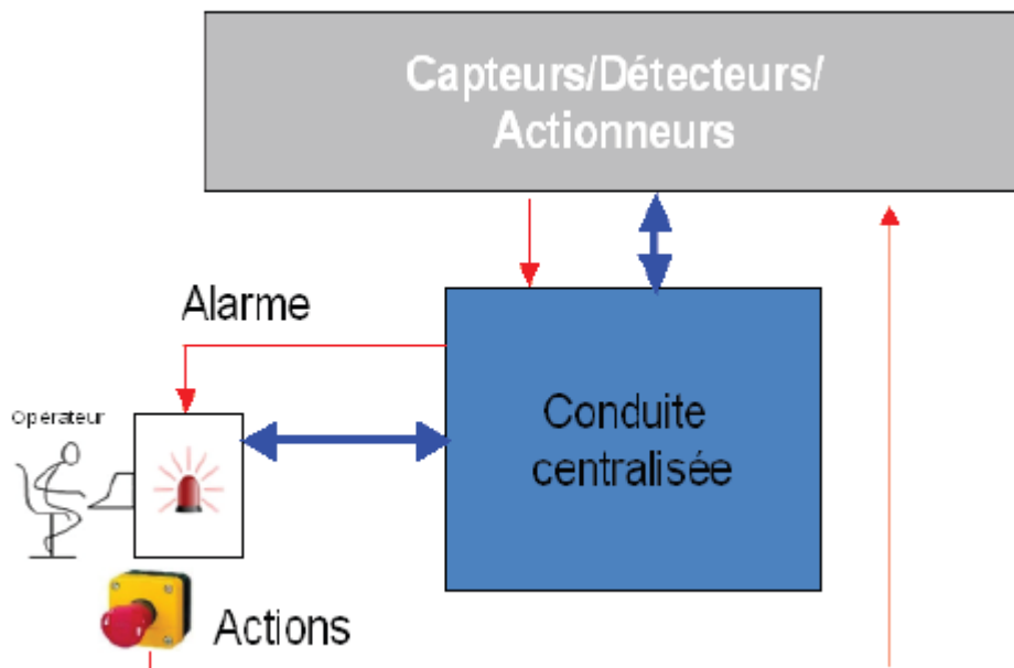
Figure 5. Alarmes qui passent par le système de conduite centralisé avec actions indépendantes.
