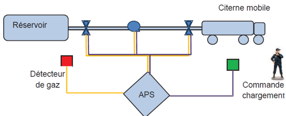
Figure 14. MMRIS avec automate non dédié exclusivement à la sécurité.
