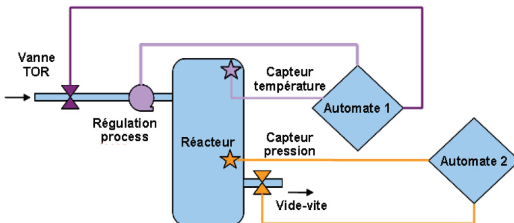
Figure 15. Principe de l'événement initiateur avec vanne TOR à l'amant.
