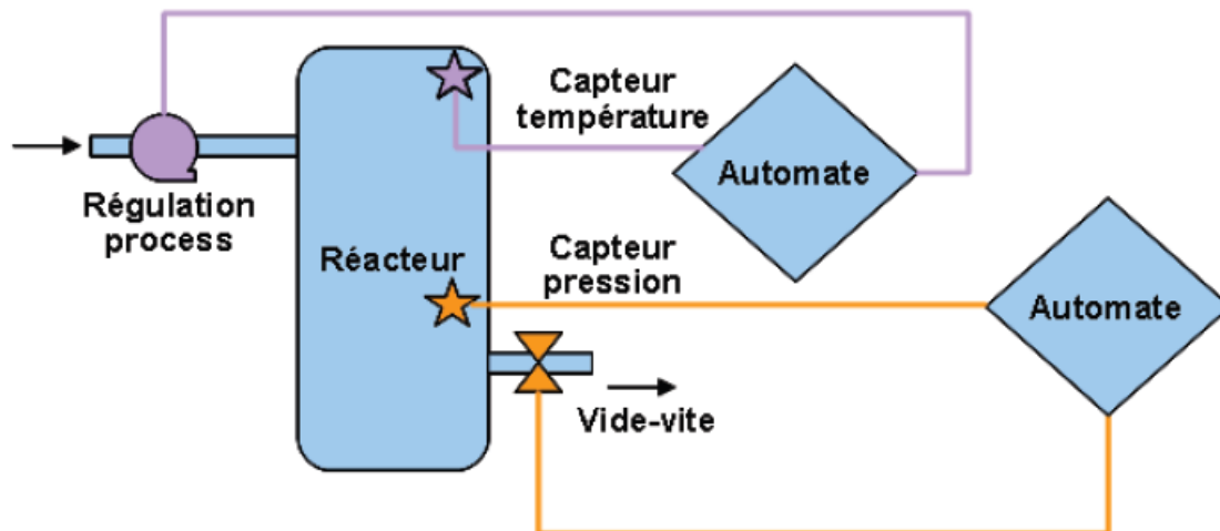
Figure 1. Principe de l'événement initiateur
