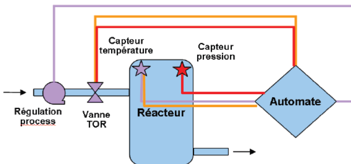
Figure 16. Chaînes avec un automate commun
