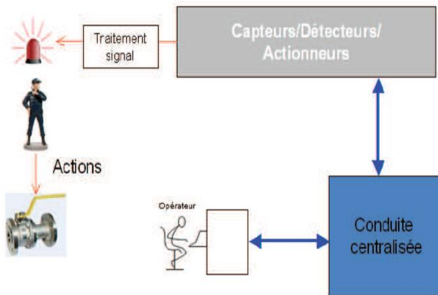
Figure 9. Alarmes, traitement et actions indépendantes du système de conduite centralisé.
