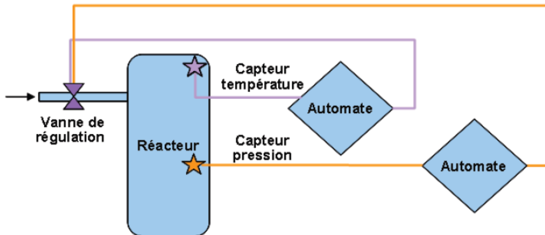
Figure 13. MMRIS, avec actionneur, utilisé pour la conduite du procédé.
