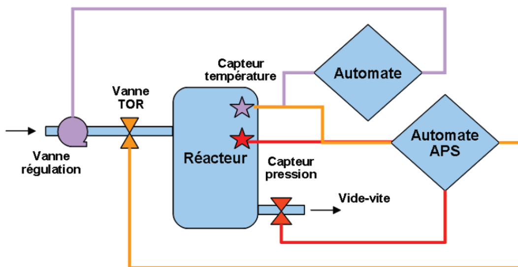
Figure 17. Principe de Chaînes avec Indépendance des MMRIS
