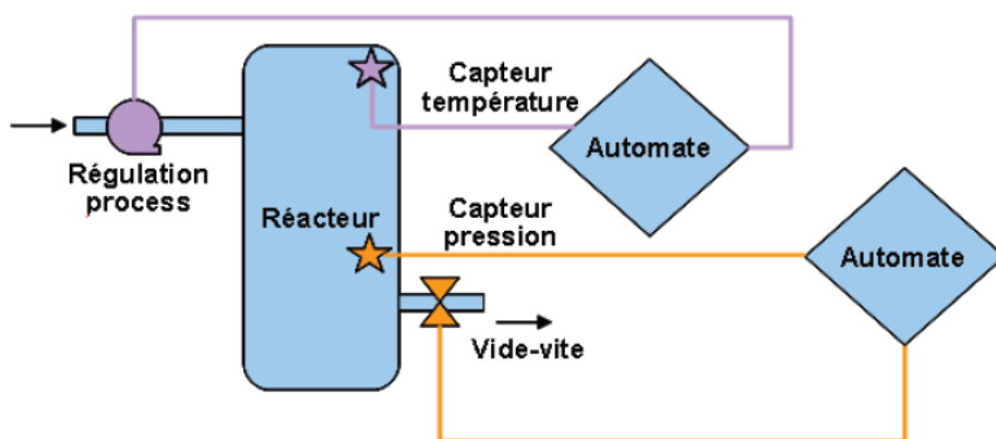
Figure 12. Les MMRIS constituées d'éléments dédiés à la sécurité.
