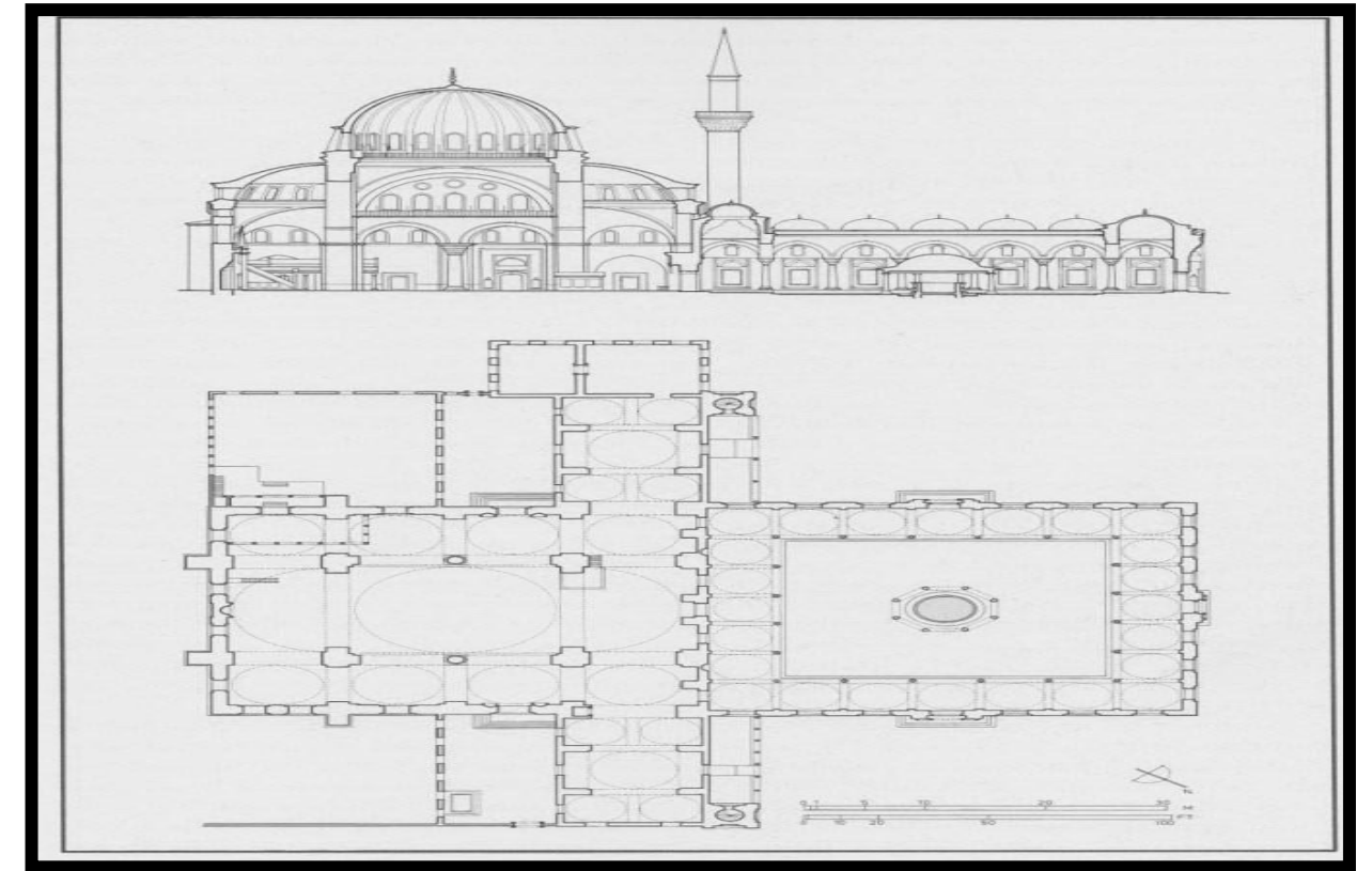
Plan et coupe de la mosquée
