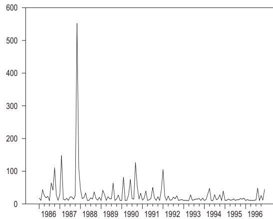
الشكل رقم (14): التباين الشرطي IGARCH(1,1)
