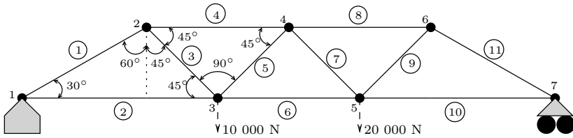
Figure 3.2 – Membrures et rotules d'une ferme
