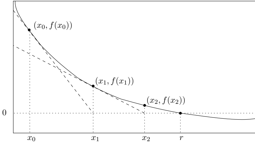
Figure 2.4 – Interprétation géométrique de la méthode de Newton
