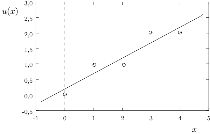
Figure 5.18 – Krigage cubique : effet pépité avec w_i = 10^5
