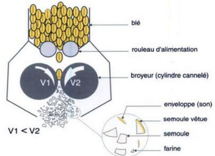
Principe de fonctionnement d'un broyeur à cylindre
