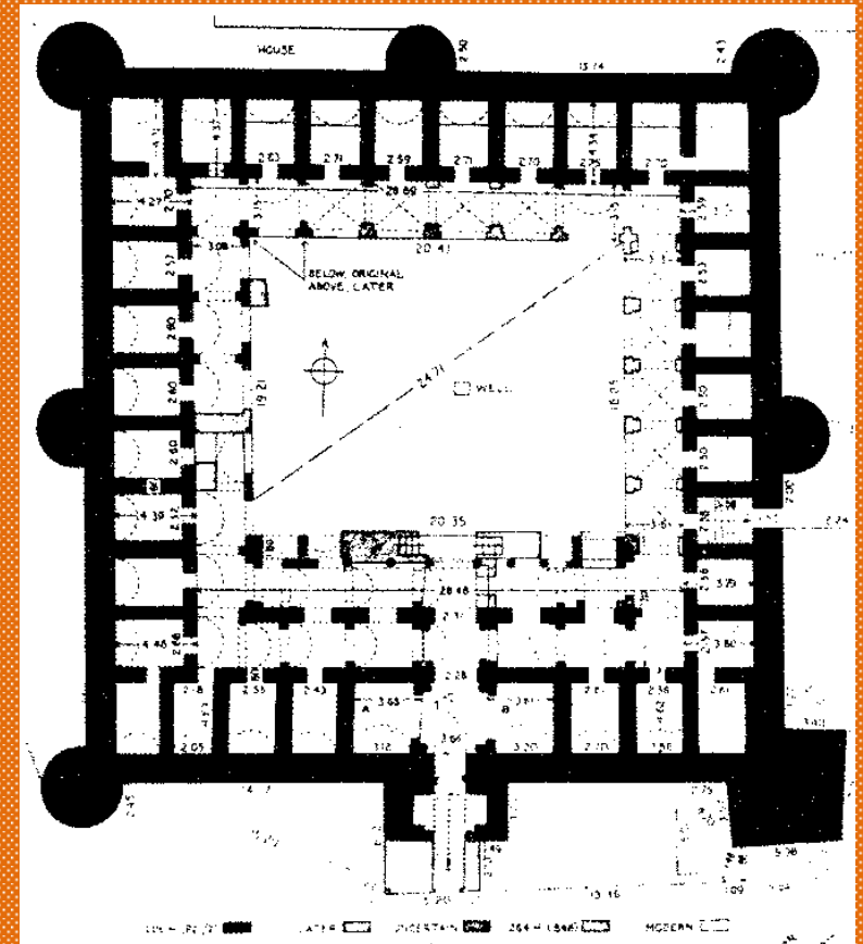
مخطط رباط المنستير الطابق الأرضي
