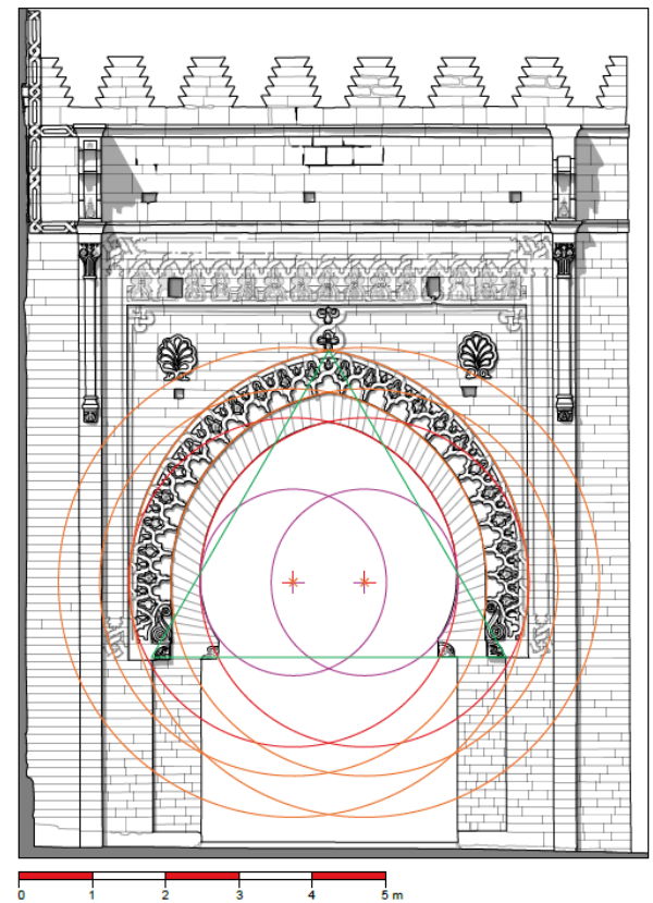
Figure 28. Schéma directeur de la façade intérieure de la porte d'aparat de Šālla (© Les auteurs).
