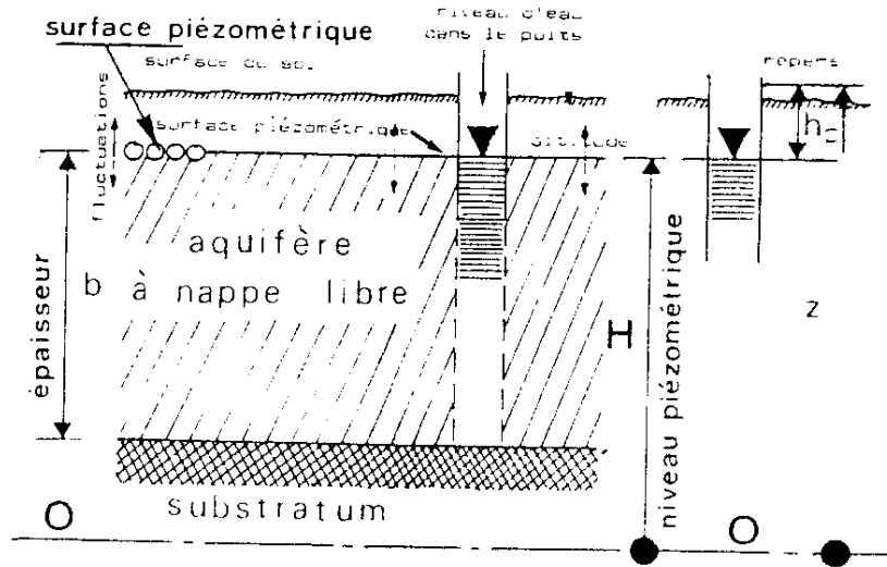
Fig n°01 : Aquifère à nappe libre
