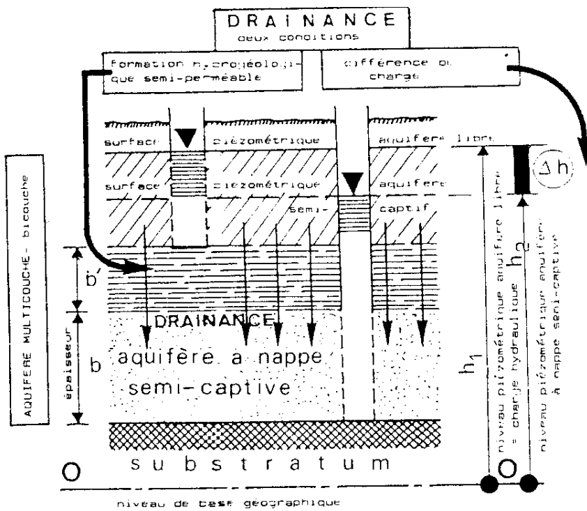
Fig n°03 : Aquifère à nappe semi- captive
