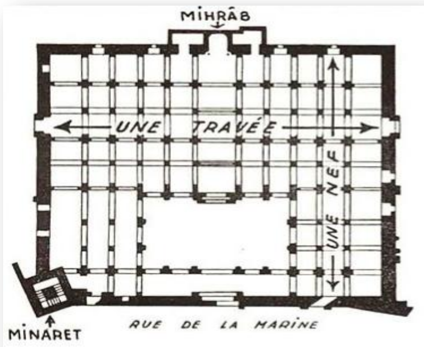
Plan de la grande mosquée d'Alger
