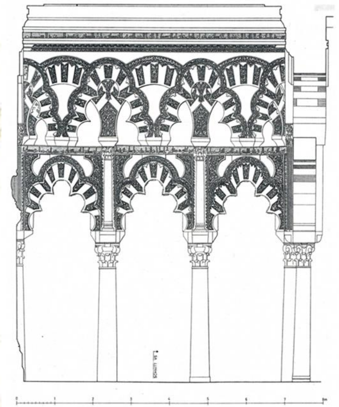
Fig. 7- Córdoba, Gran mezquita, sala de oraciones, sistema de arcos entrecruzados VSS (situación: v. fig. 4; Ev. 1968, hoja VSS D, 1: 50.
