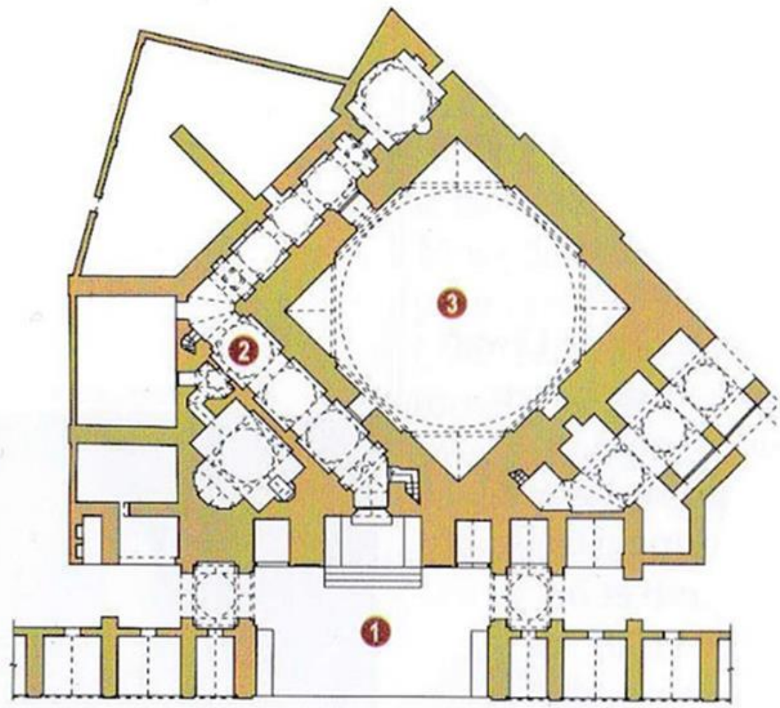
Plan de la mosquée Lotfollâh.
